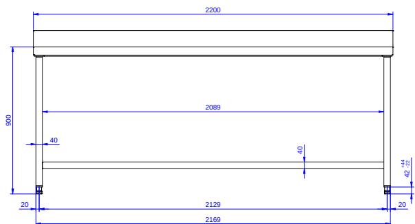
Zepředu
